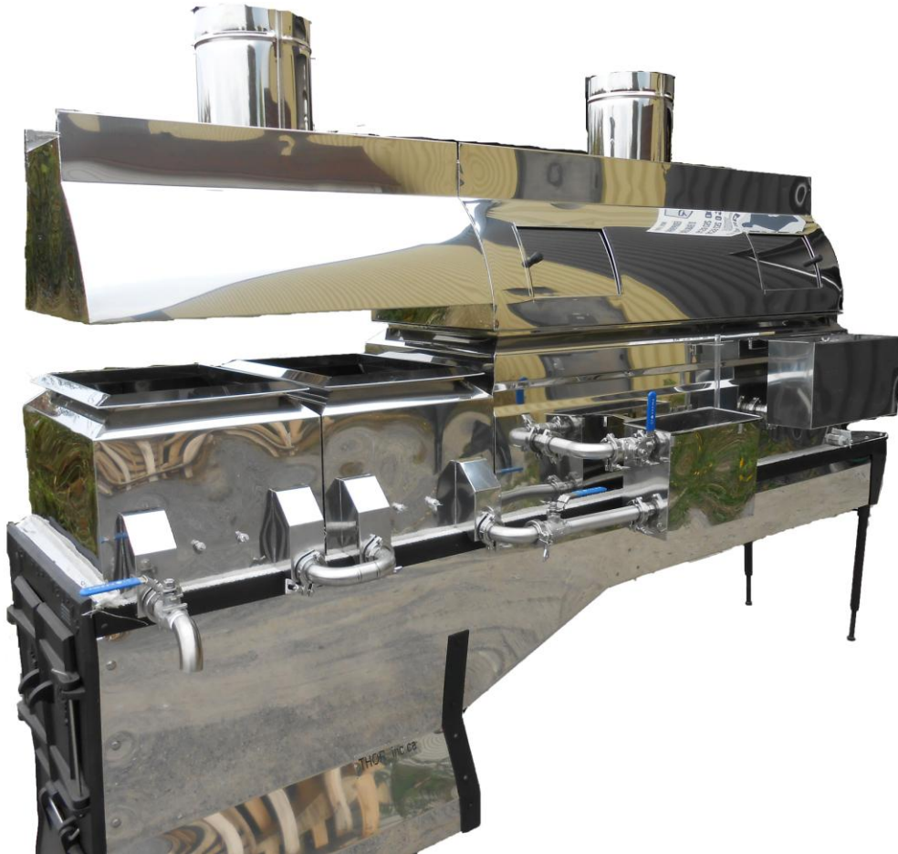
CLASIQUE WOOD FIRE EVAPORATOR
